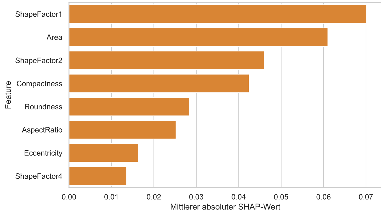
Globale SHAP-Wichtigkeit des Random Forest
